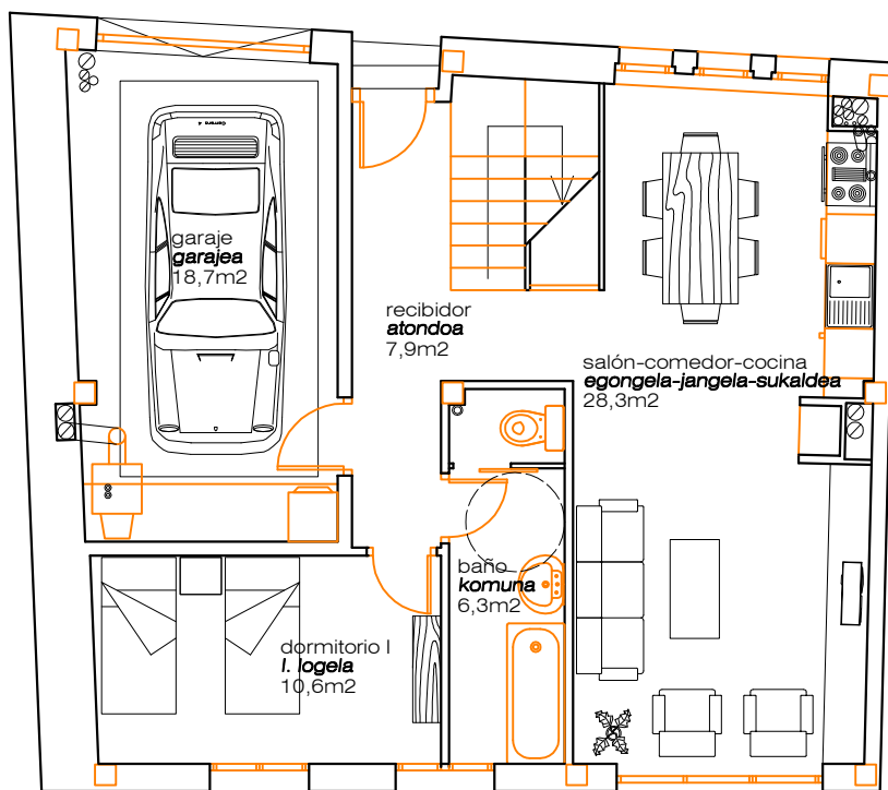
Bigarren solairua Planta segunda (nivel III)
