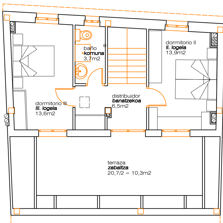
Hirugarren solairua Planta tercera (nivel IV)
